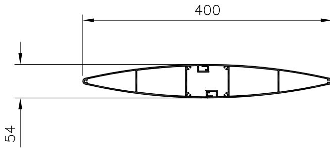
MF400 FIN BLADE EXTRUDED ALUMINIUM
