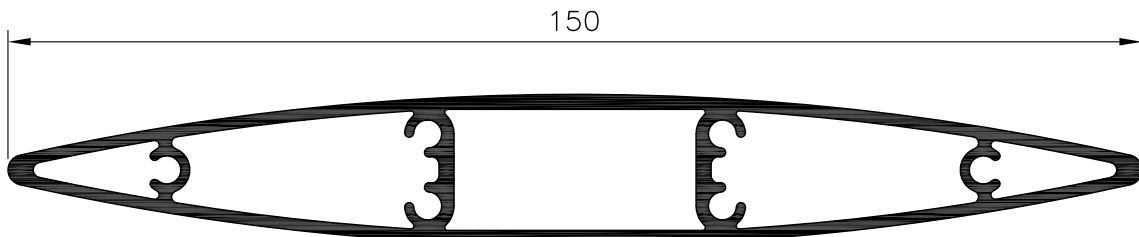
MF150 BLADE
